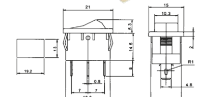
PRZEŁĄCZNIK MK1011
