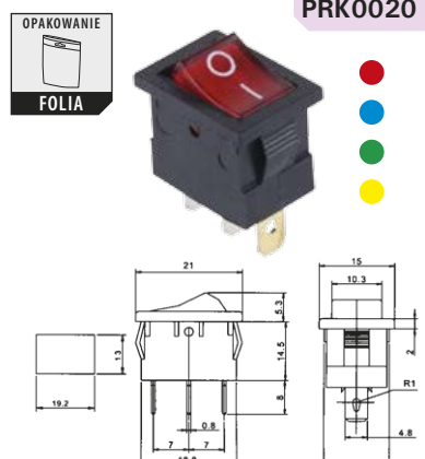
PRZEŁĄCZNIK MK1011
