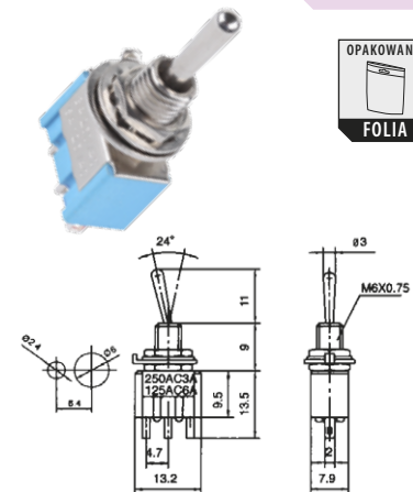
PRZEŁĄCZNIK MTS 100
