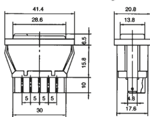
PRZEŁĄCZNIK ASW-02D
