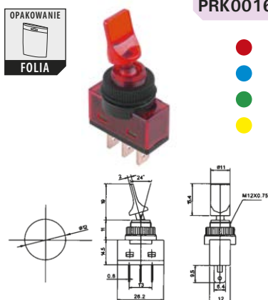
PRZEŁĄCZNIK ASW-14D
