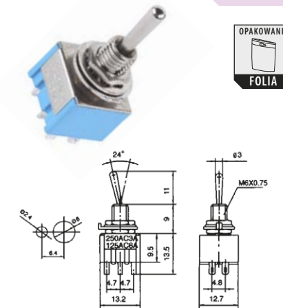
PRZEŁĄCZNIK MTS 200
