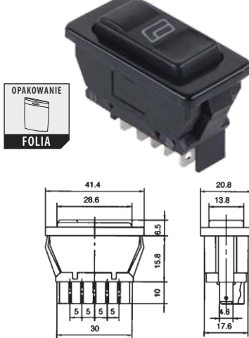
PRZEŁĄCZNIK ASW-02D
