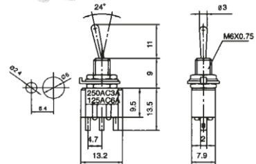
PRZEŁĄCZNIK MTS 100
