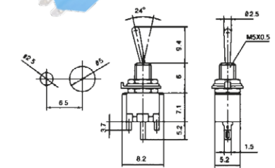
PRZEŁĄCZNIK SMTS 100
