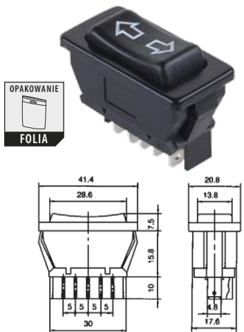
PRZEŁĄCZNIK ASW-01
