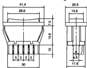
PRZEŁĄCZNIK ASW-01
