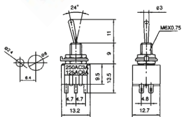
PRZEŁĄCZNIK MTS 200
