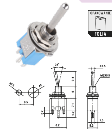
PRZEŁĄCZNIK SMTS 100
