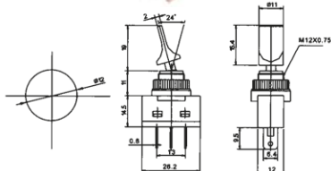
PRZEŁĄCZNIK ASW-14D
