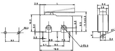
PRZEŁĄCZNIK MSW-12B
