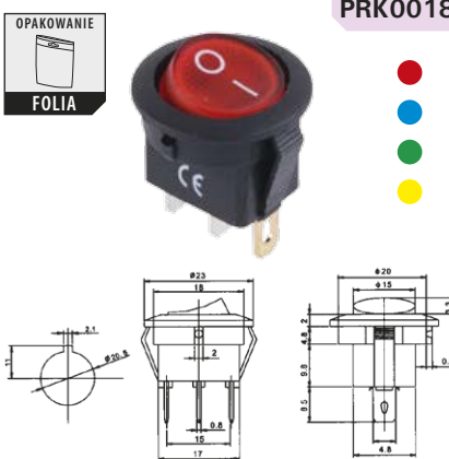
PRZEŁĄCZNIK IRS-101-8C/D
