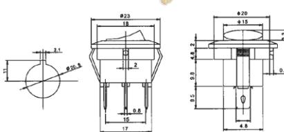
PRZEŁĄCZNIK IRS-101-8C/D
