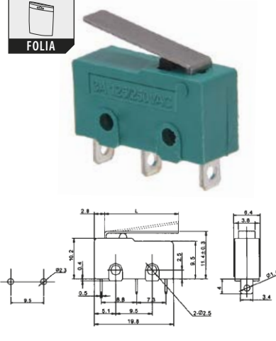
PRZEŁĄCZNIK MSW-12B
